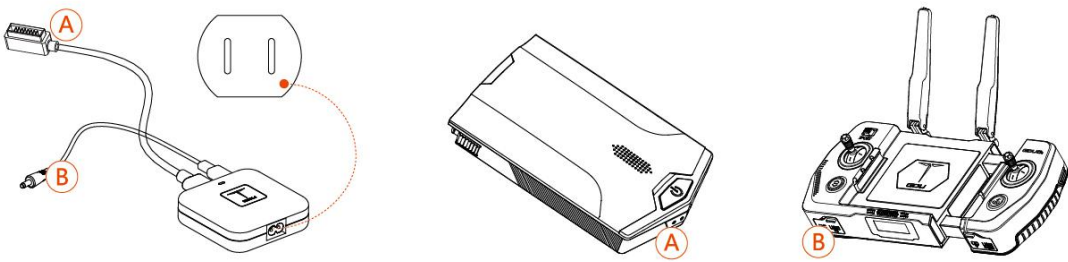
输入电压：100~240V 充电时长：A+B小于2.5小时
